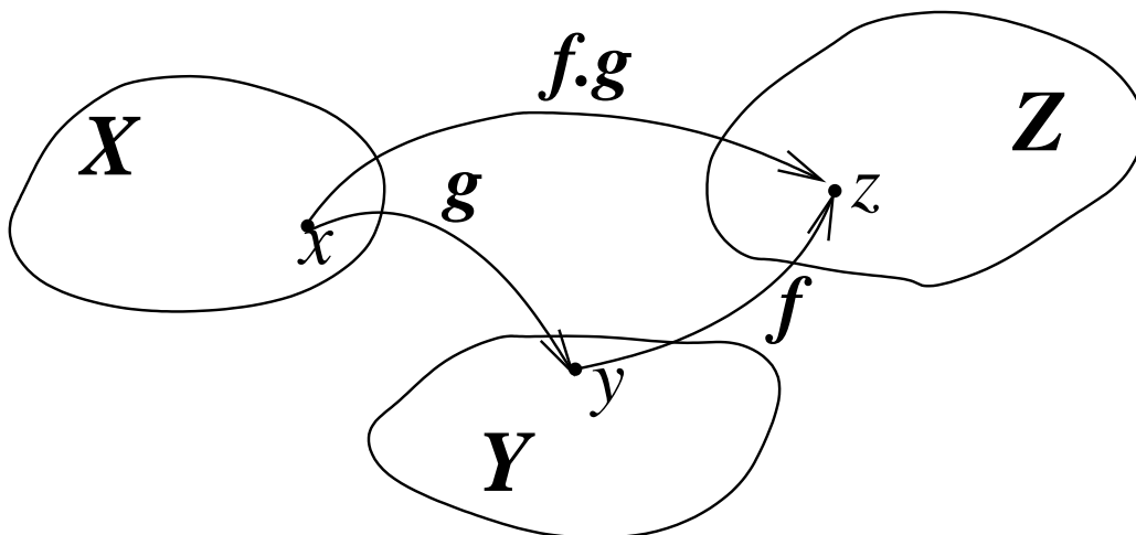
Рис. 1. Композиция функций
